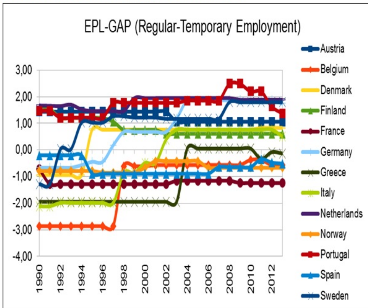
Fig. 1 - Andamento dell'indice EPLgap in Europa, 1990-2013
